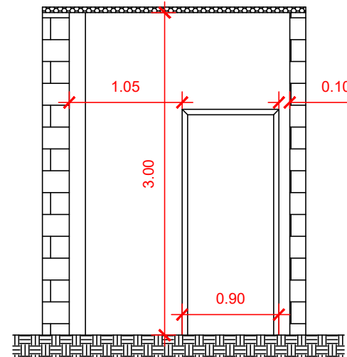
CORTE A-A
