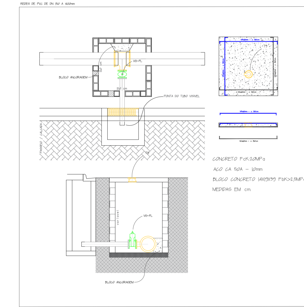
DETALHES DA REDE ESC: 1:50
