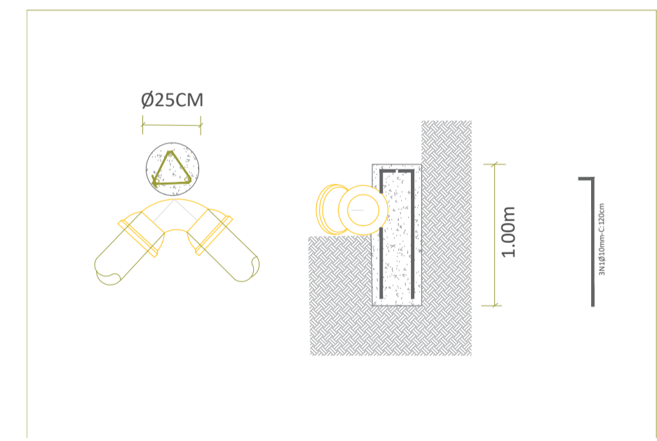
DETALHES DA BROCAS DE ANCORAGEM S/ESC
