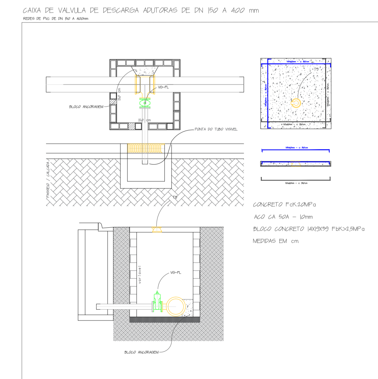
DETALHES DA REDE ESC: 1:50
