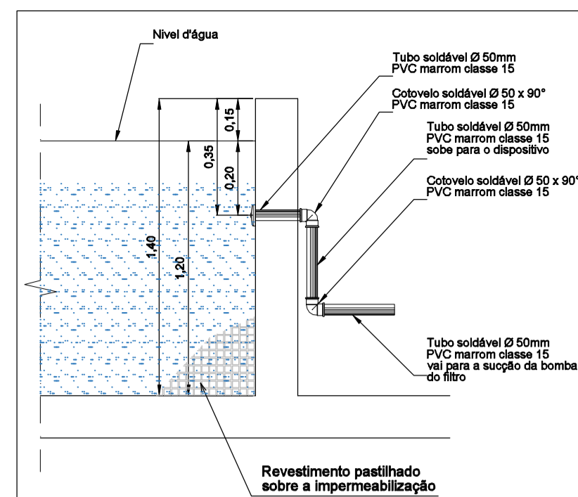
Detalhe construtivo Aspiração
