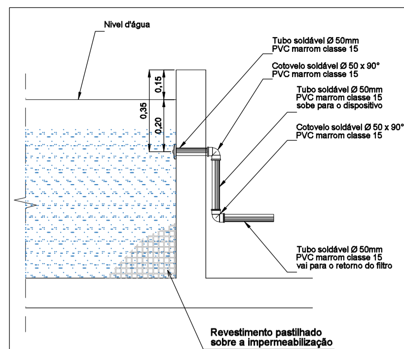
Detalhe construtivo Retorno de água filtrada
