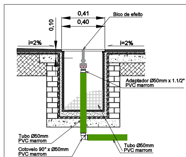
Detalhe construtivo Bico de efeito
