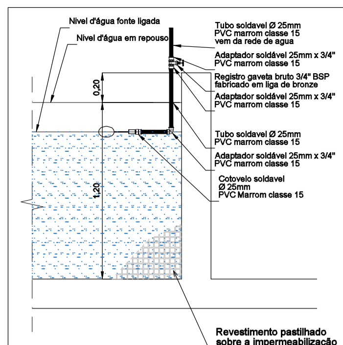
Detalhe construtivo Alimentação de água
