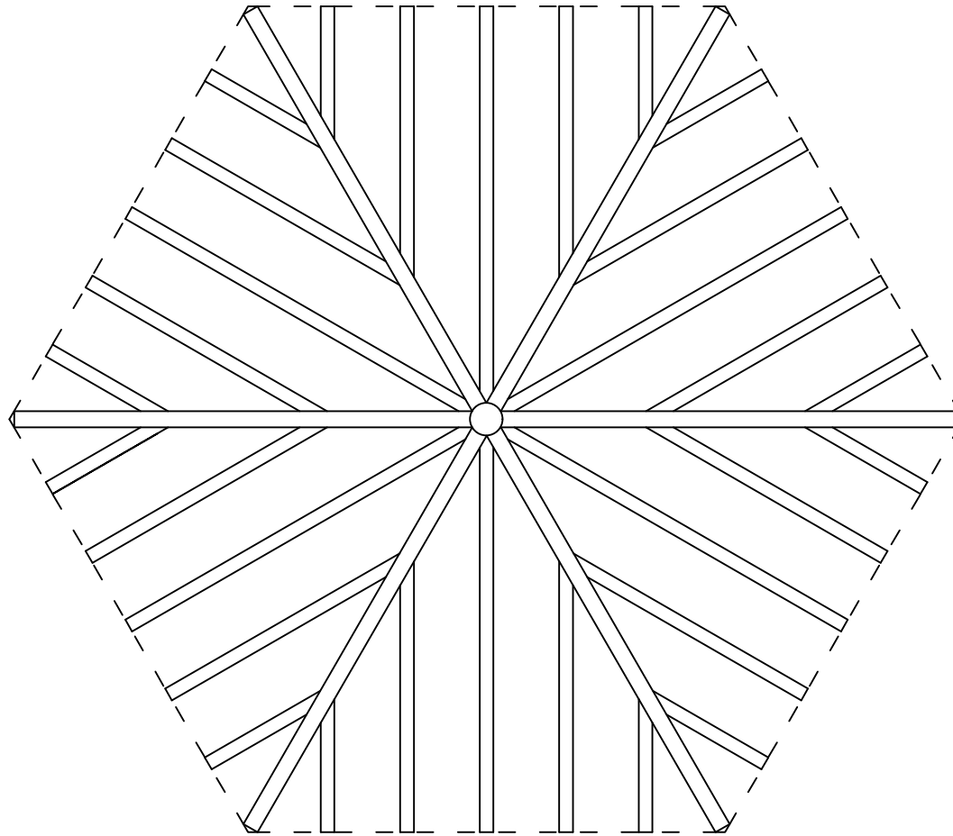
DETALHE CAIBRAMENTO ESCALA 1:50
