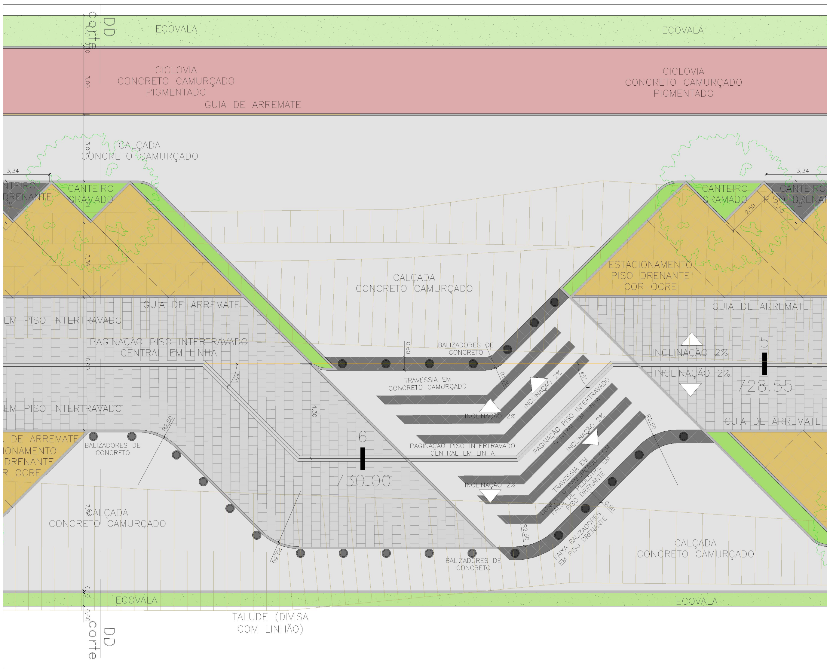
DETALHE: TRAVESSIA ESCALA 1:100
