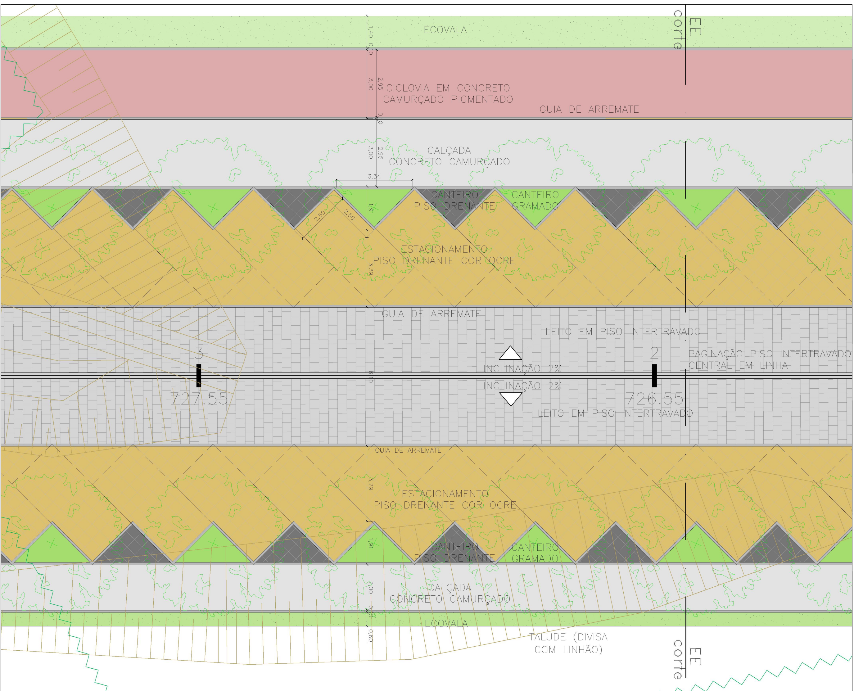
DETALHE: PADRÃO ESCALA 1:100
