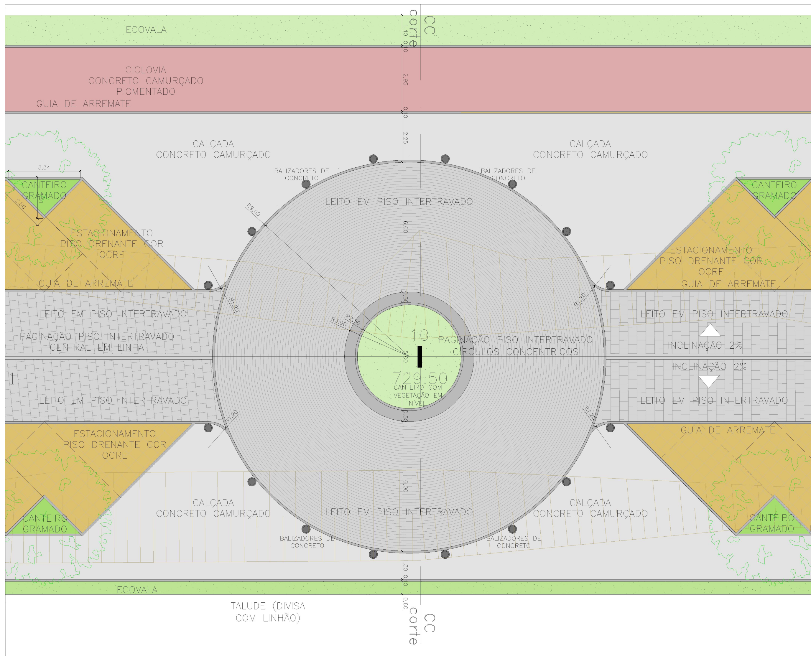
DETALHE: DISPOSITIVO DE RETORNO ESCALA 1:100
