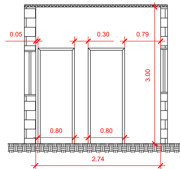
CORTE A-A
