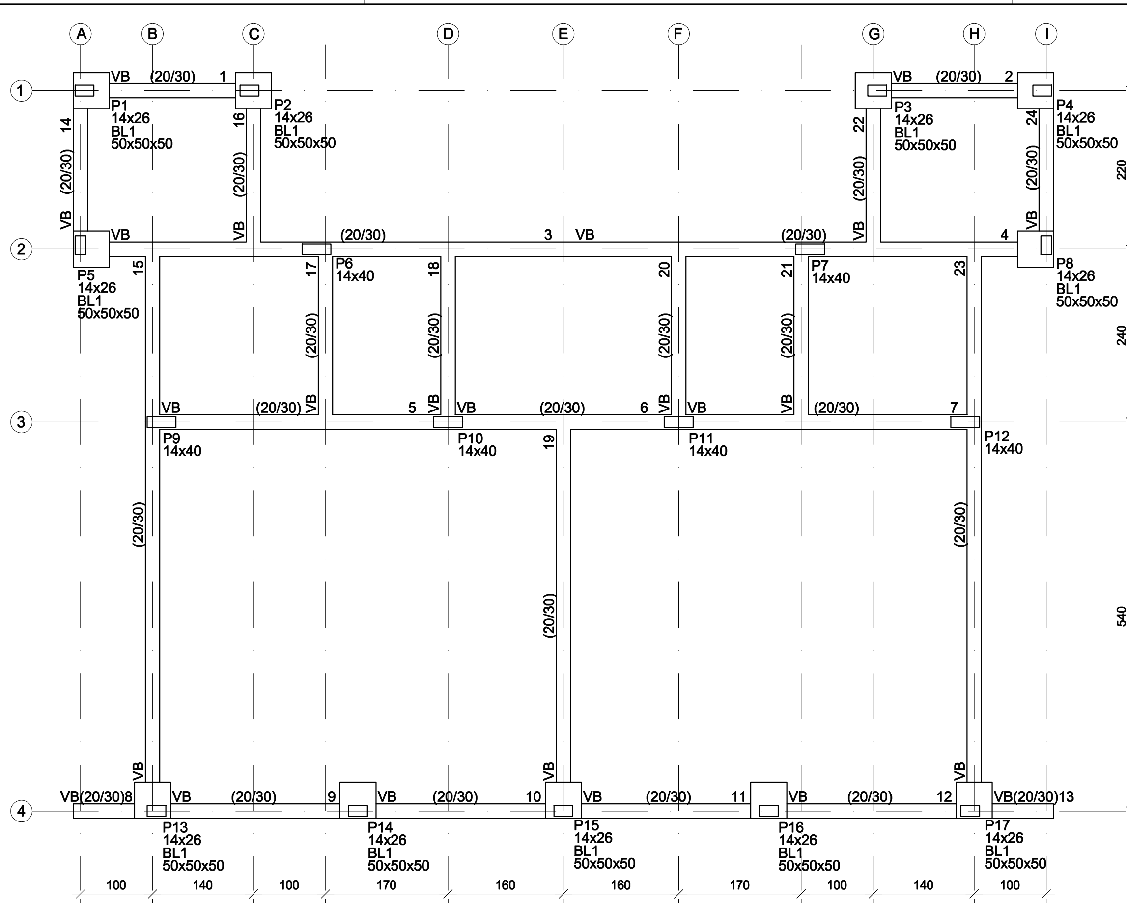
FORMA DE FUNDAÇÃO ESC. 1:50
