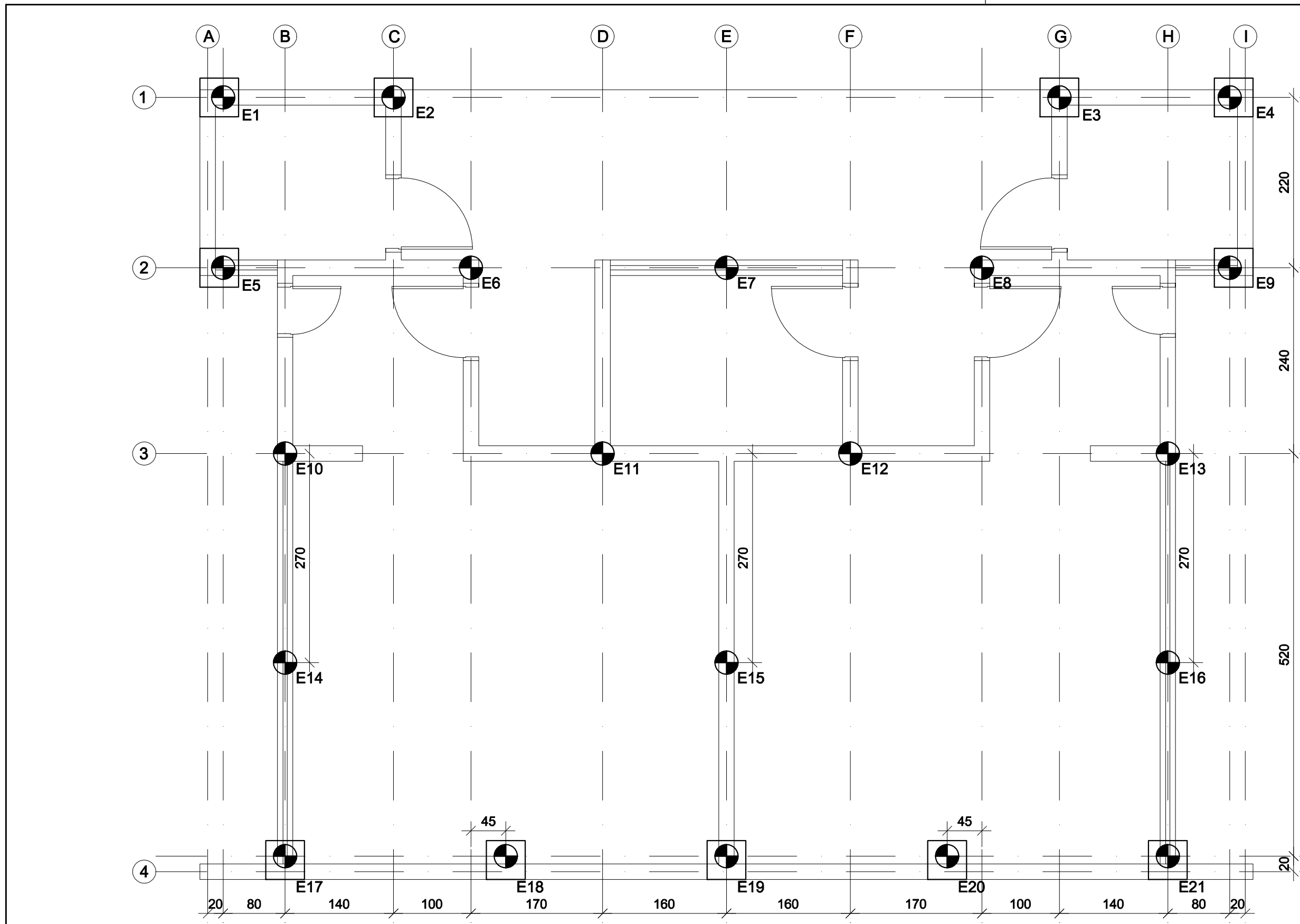
LOCAÇÃO DE ESTACAS ESC. 1:50
