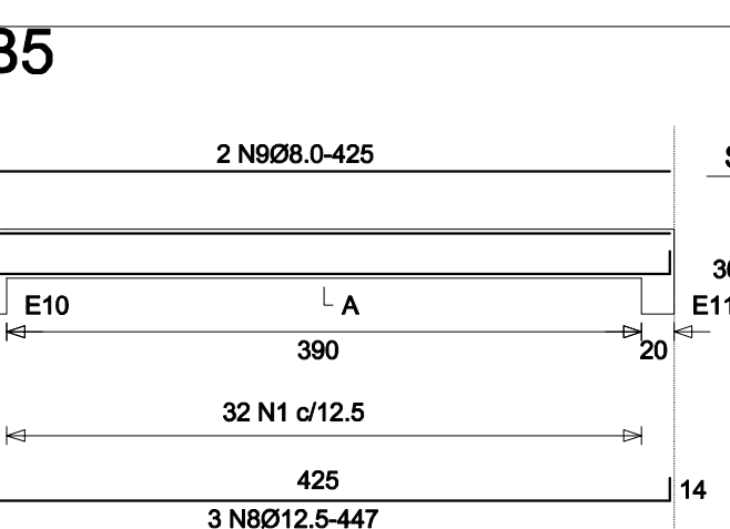
FORMA DE FUNDAÇÃO ESC. 1:50
