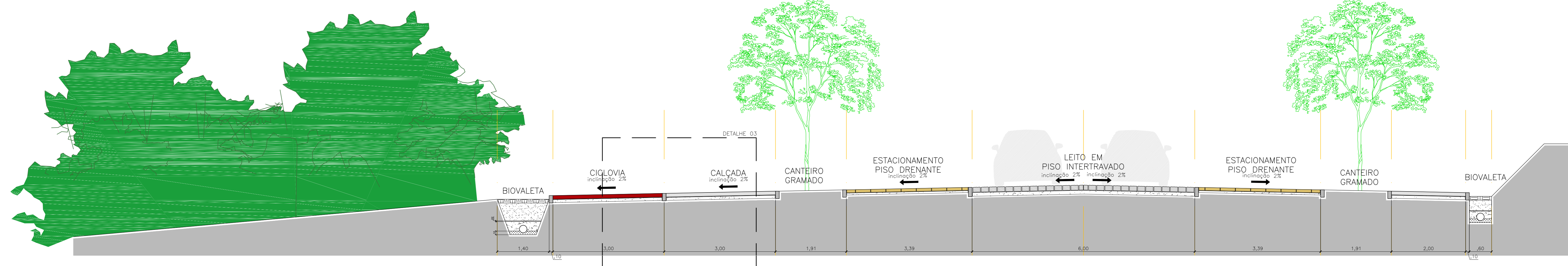
CORTE ESTACA 2+12,30m ESCALA 1:50
