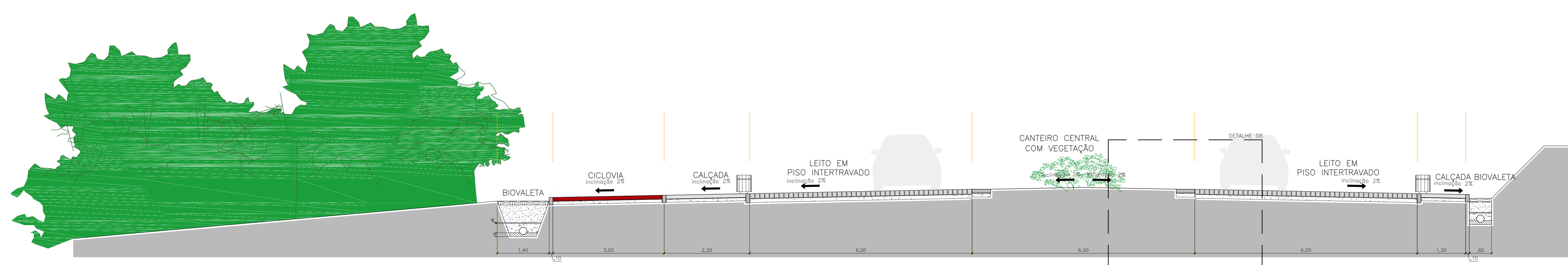
CORTE ESTACA 10+0,49m ESCALA 1:50
