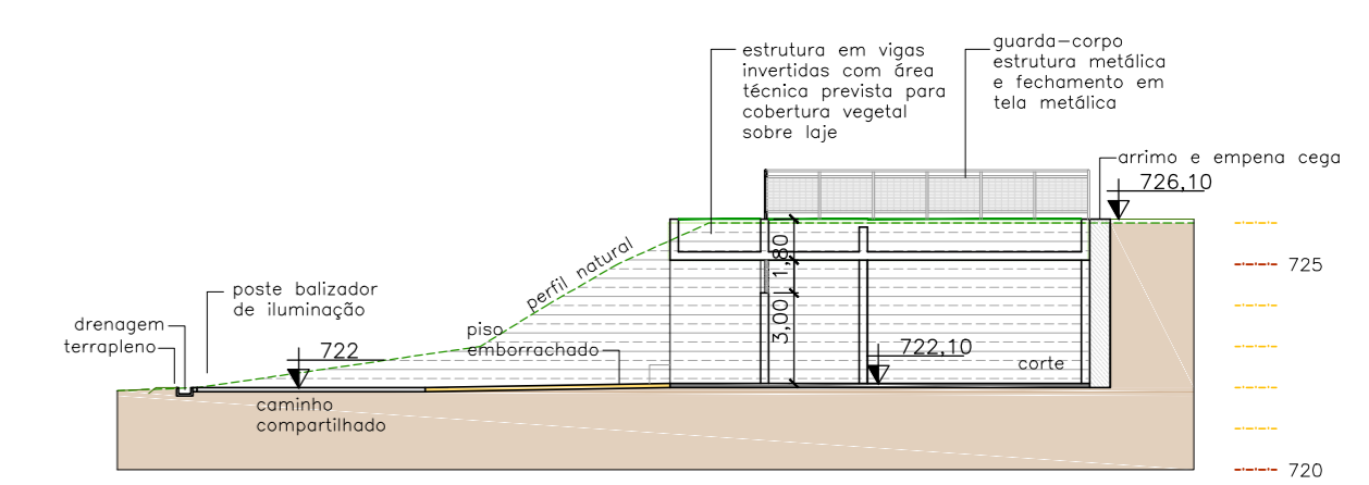
CORTE 81 escala 1:200
