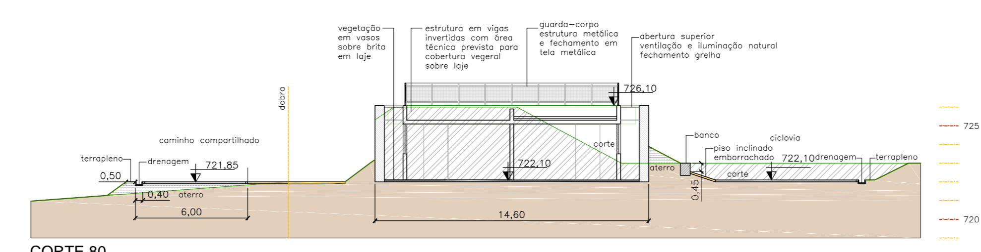
CORTE 80 escala 1:200
