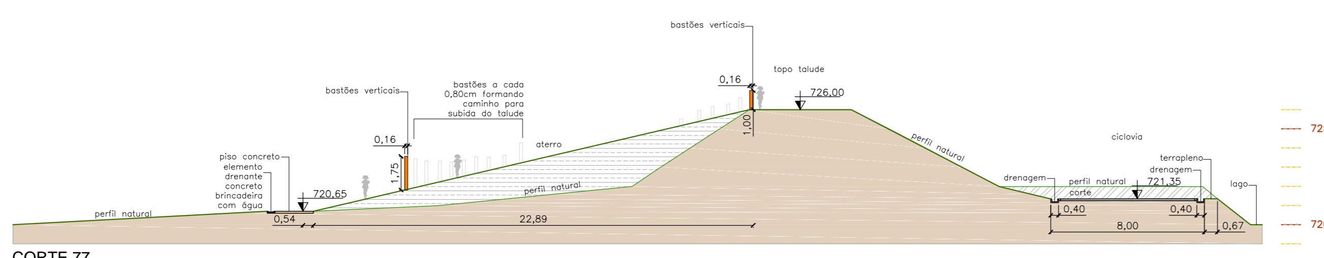
CORTE 77 escala 1:200
