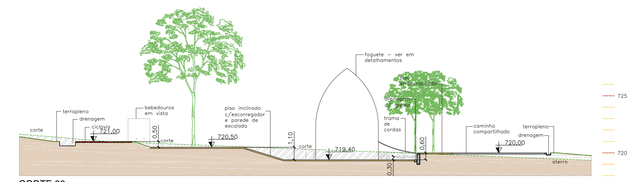
CORTE 82 escala 1:200
