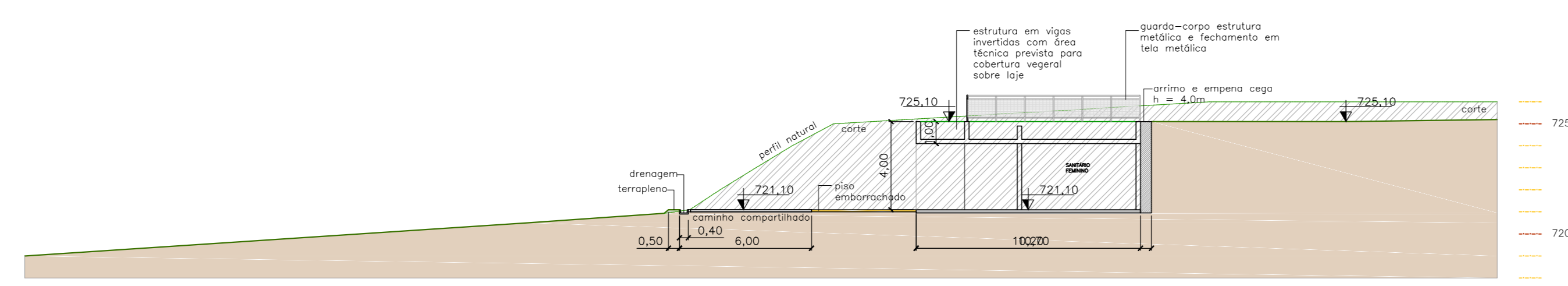
CORTE 75 escala 1:200
