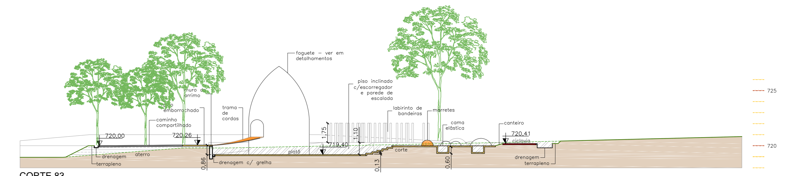
CORTE 83 escala 1:200
