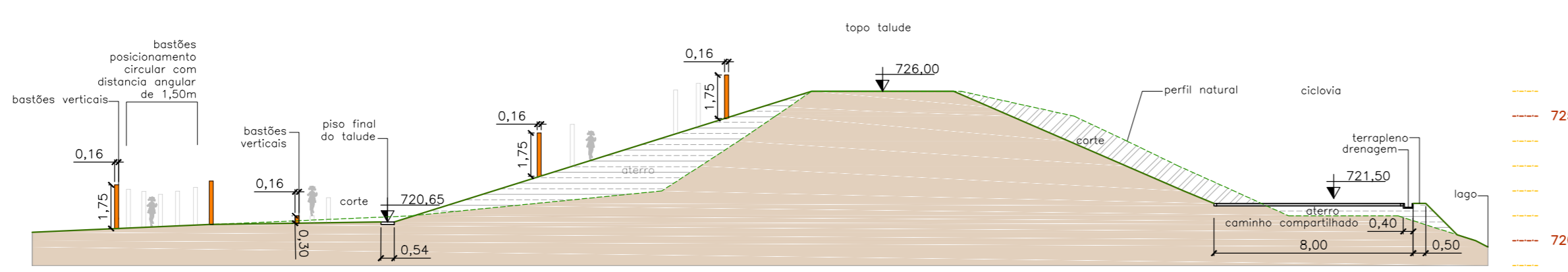
CORTE 78 escala 1:200
