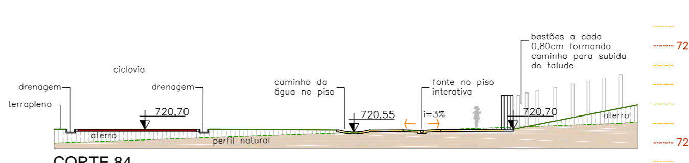
CORTE 84 escala 1:200
