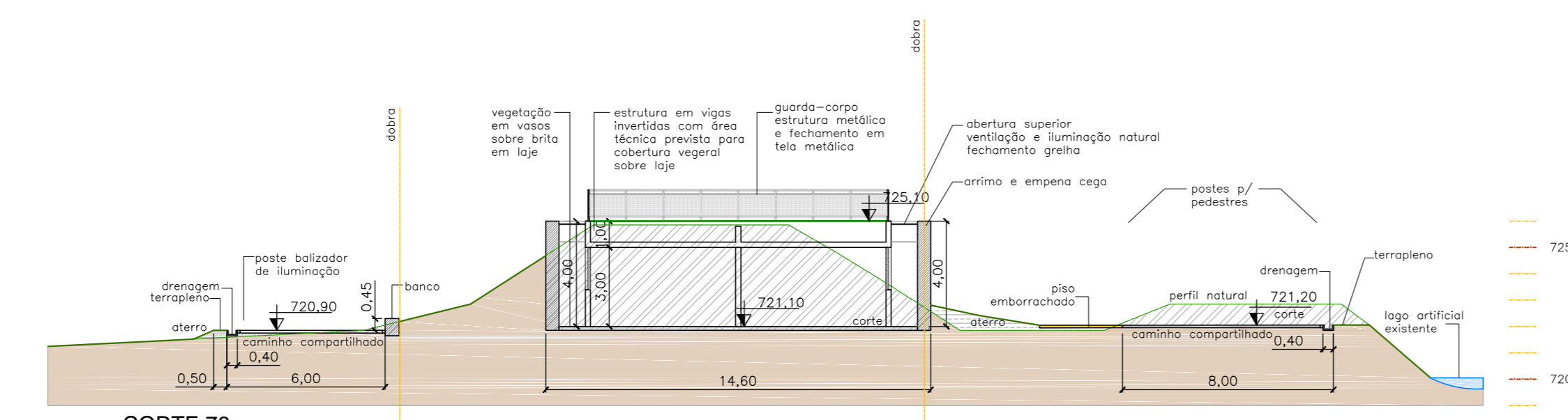
CORTE 76 escala 1:200
