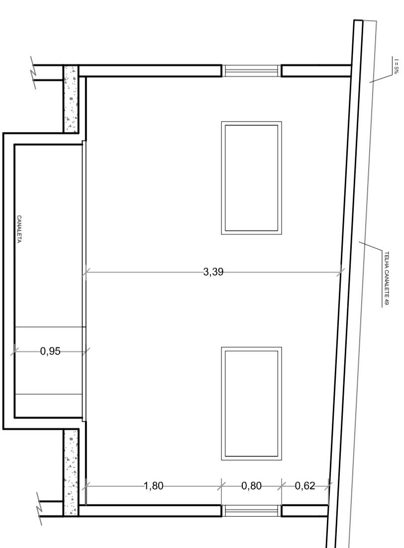
CORTÉ D-D
