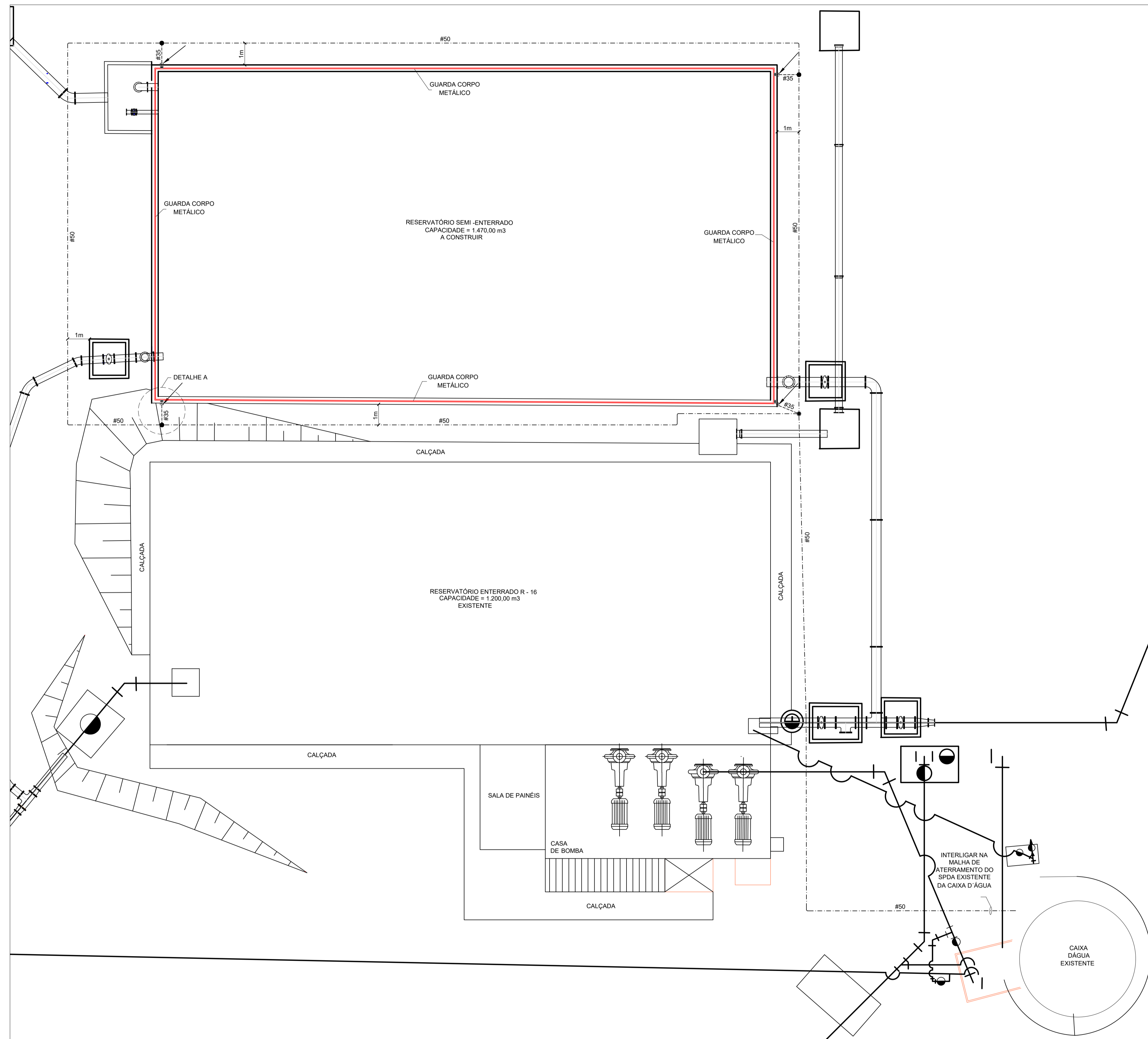
IMPLANTAÇÃO ATERRAMENTO DO GUARDA CORPO E ESCADAS DO RESERVATÓRIO ESCALA 1:100
