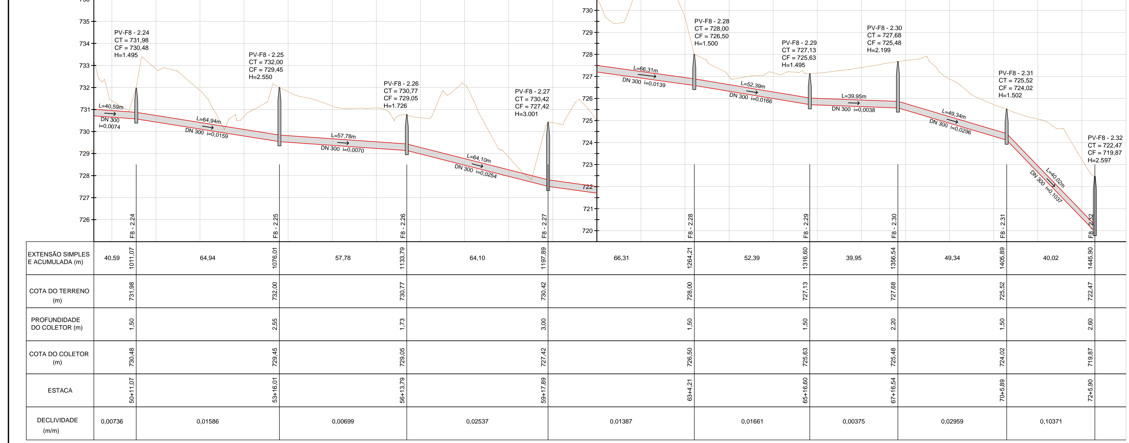
PERFIL LONGITUDINAL ESCALA: HORIZONTAL 1/1000 VERTICAL 1/100
