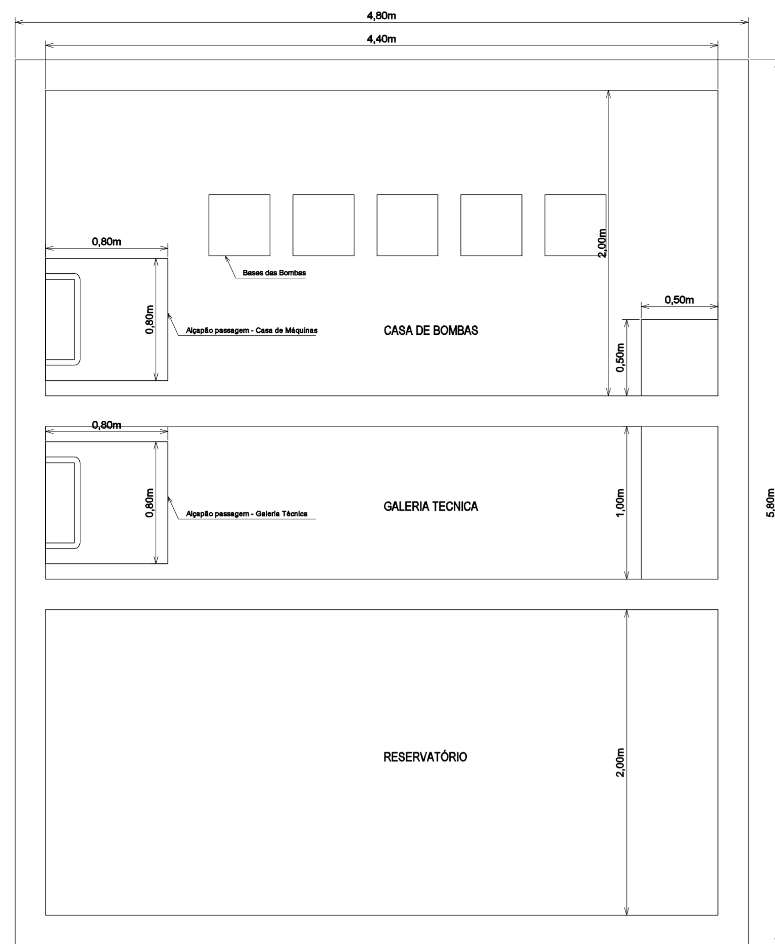
CASA DE BOMBAS PLANTA BAIXA ESC. 1/25 MEDIDAS EM METROS
