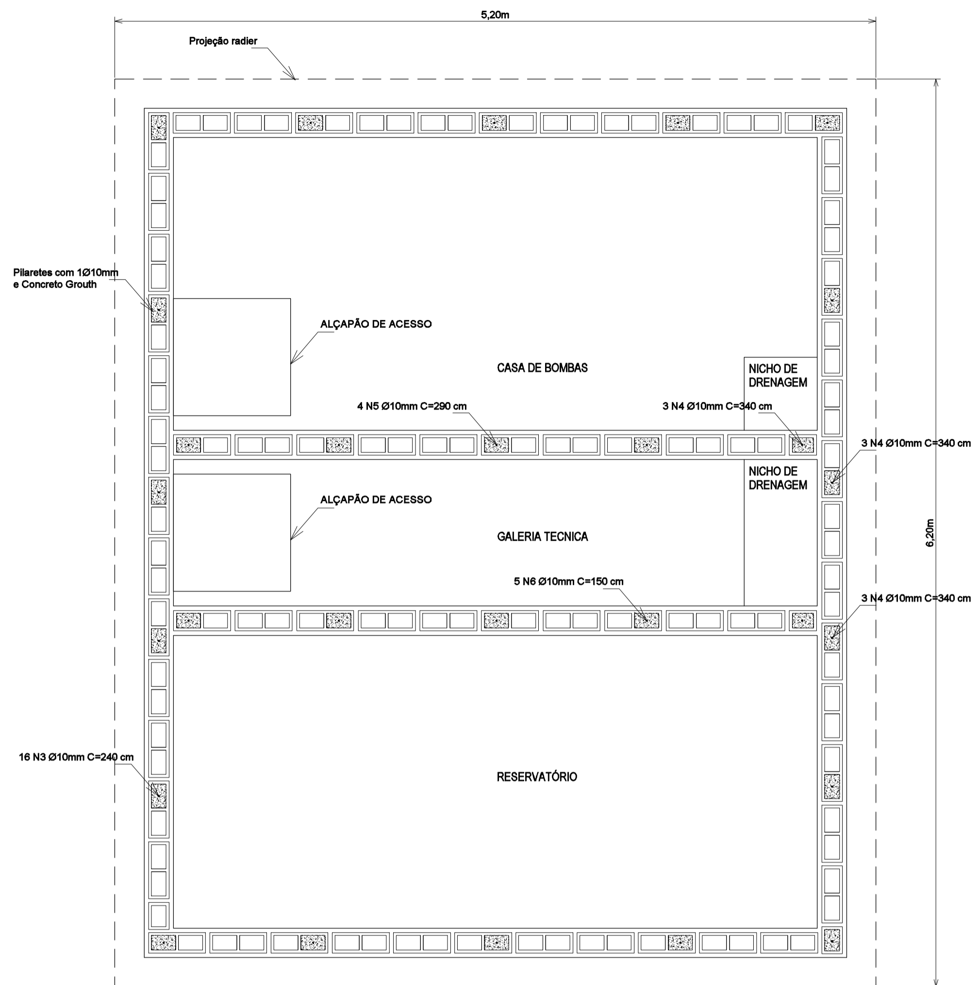
CASA DE BOMBAS FABRICAÇÃO DA ALVENARIA ESC. 1/25 MEDIDAS EM METROS
