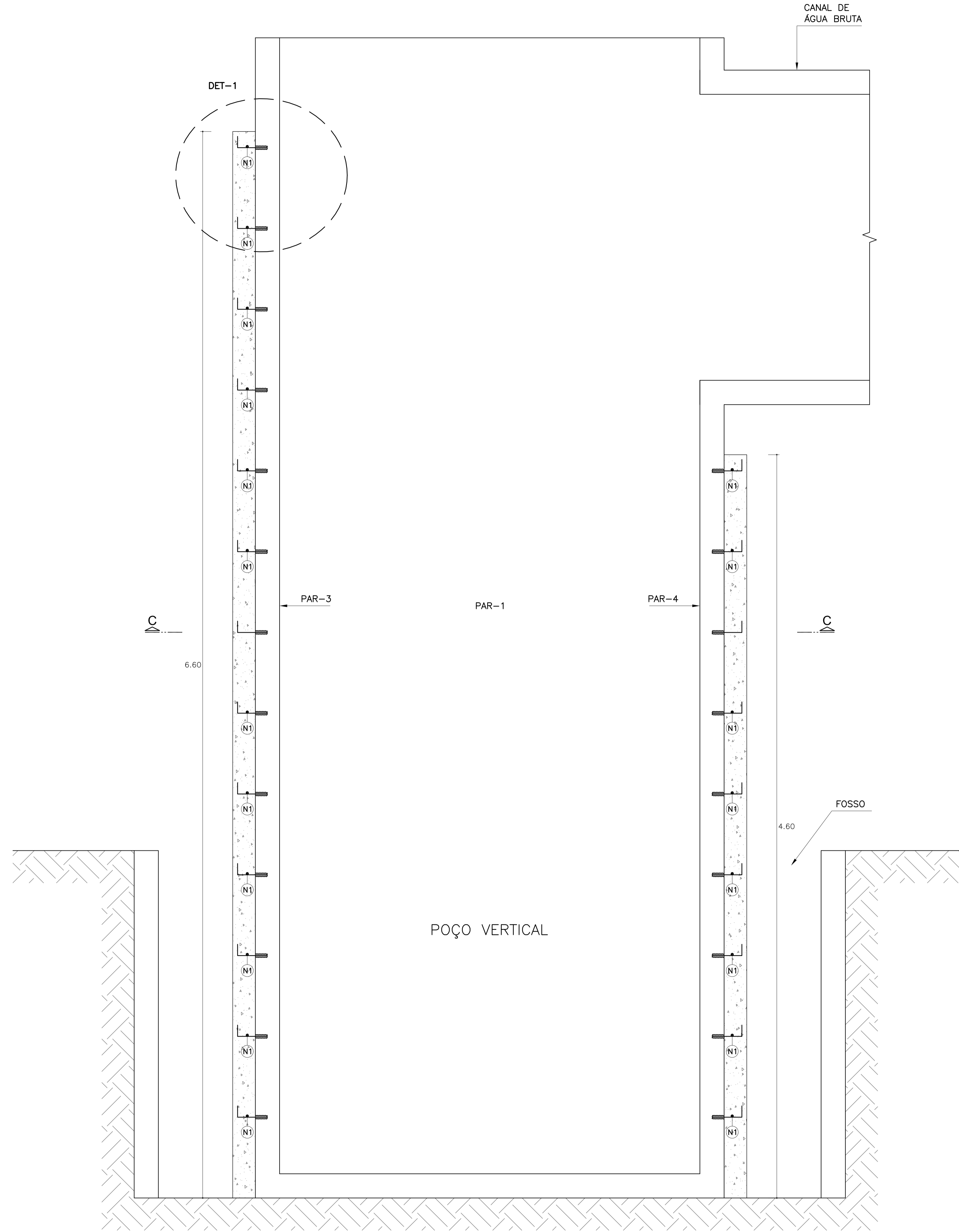
CORTE A-A Escala: 1:12,5
