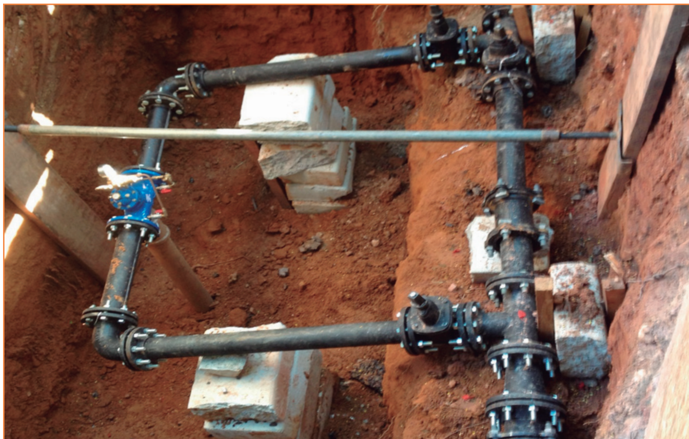
Figura 6 - Exemplo de Instalação de VRP
