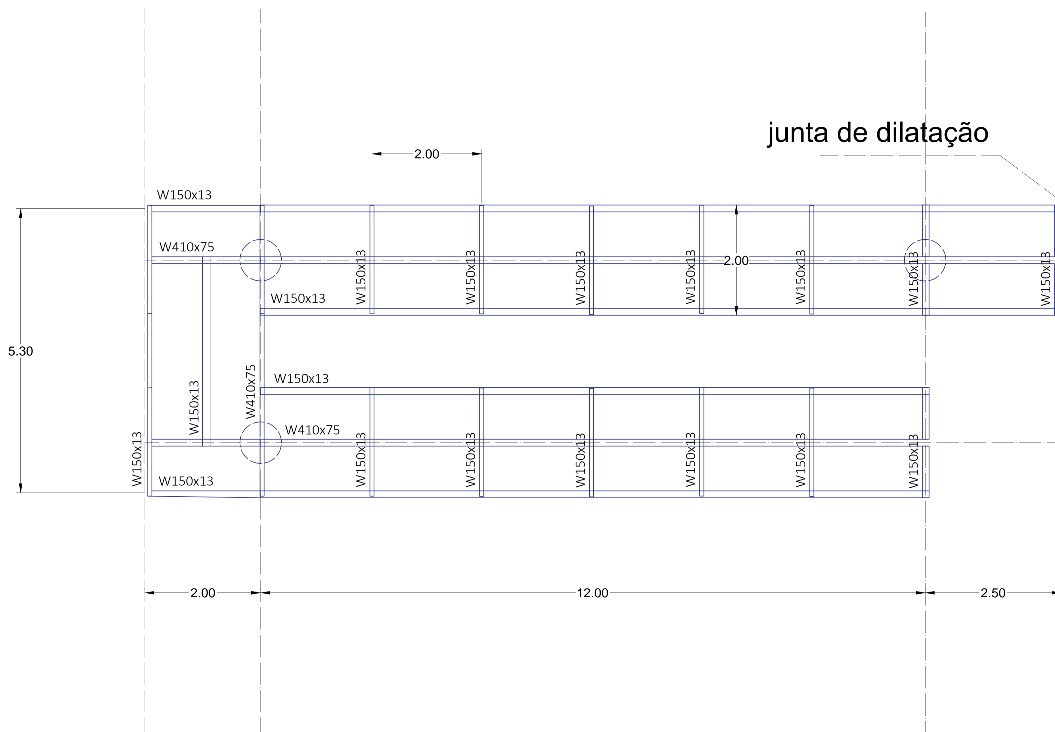
PLANTA BAIXA
