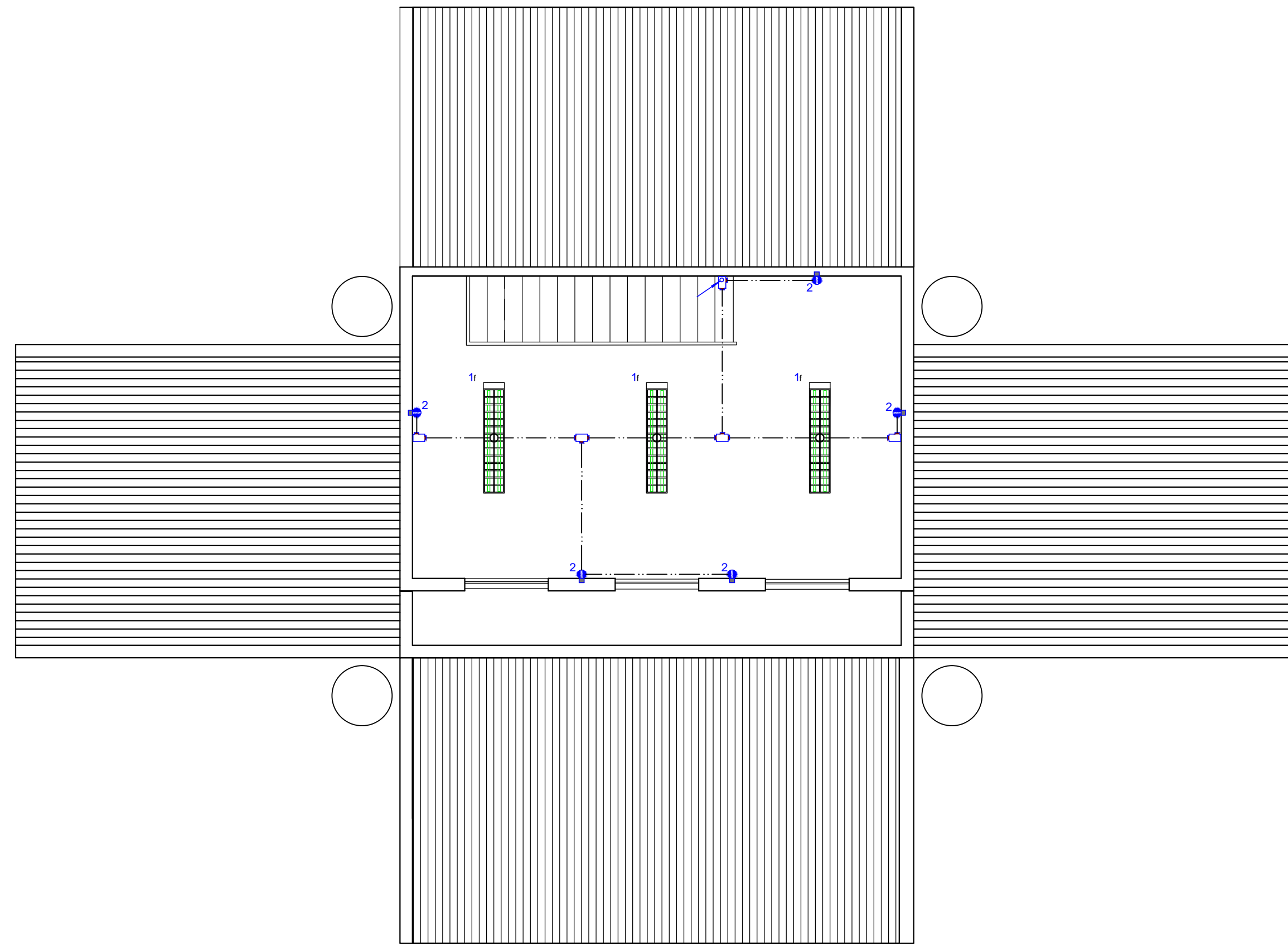
ARQUITETURA - NÍVEL= 4.65
