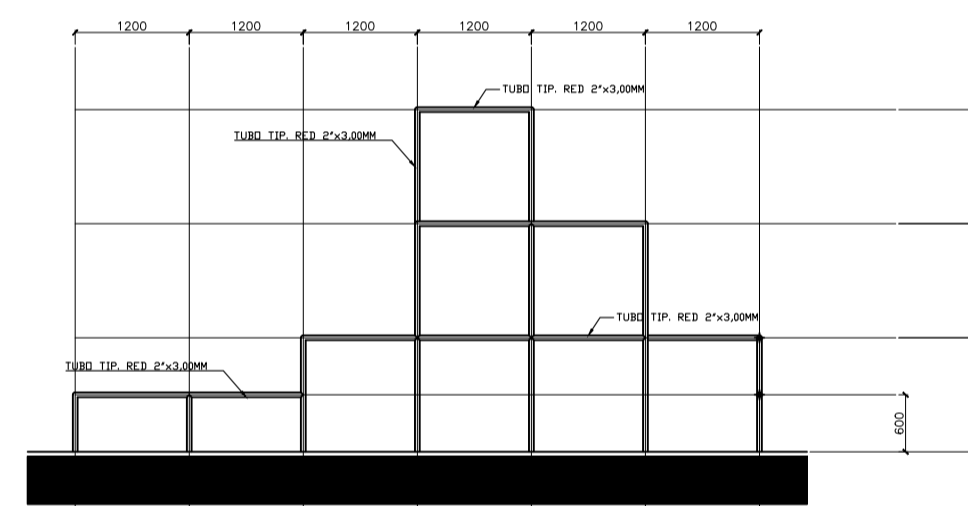
VISTA 10 ESCALA 1:75
