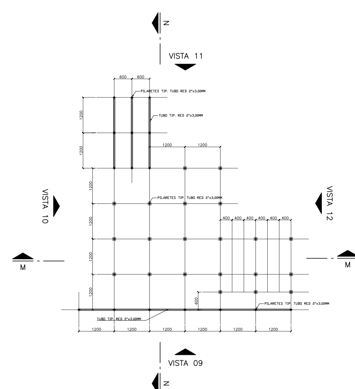
CONJUNTO 03 – Nível +0,60 ESCALA 1:75
