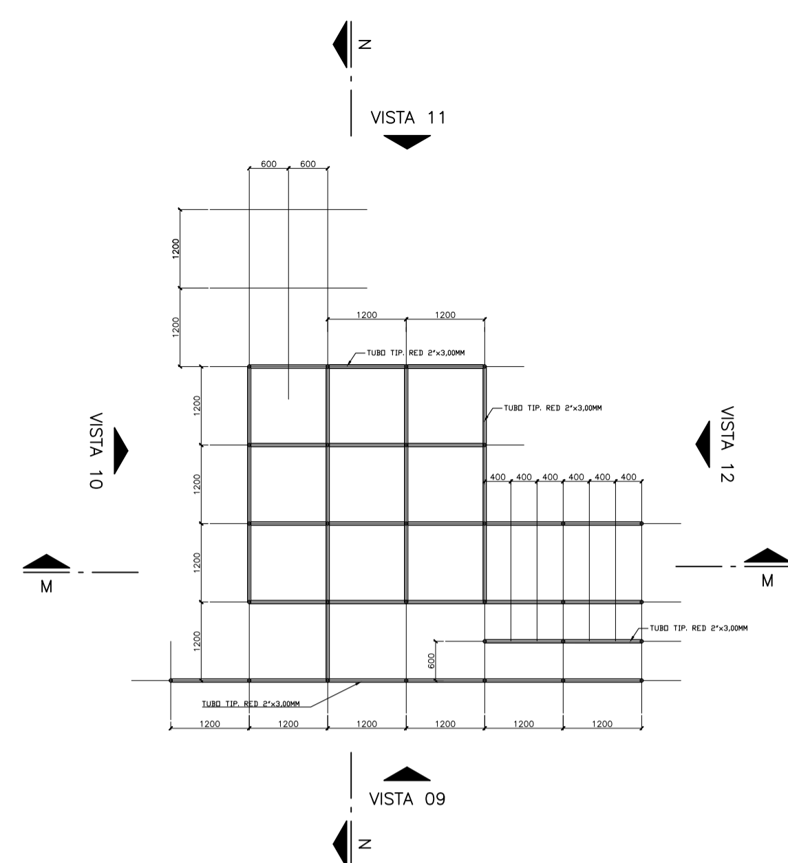
CONJUNTO 03 – Nível +1,20 ESCALA 1:75
