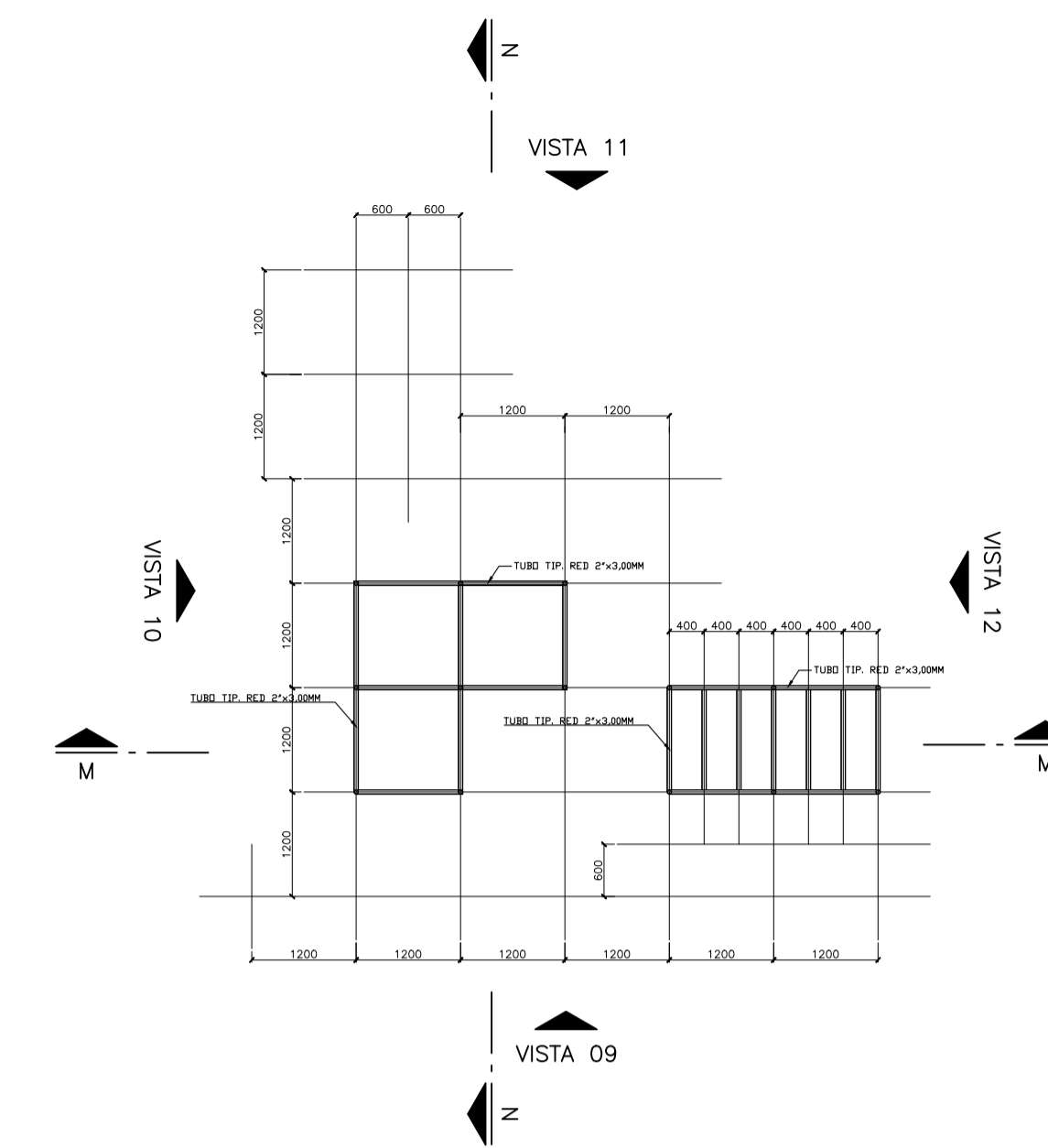
CONJUNTO 03 – Nível +2,40 ESCALA 1:75
