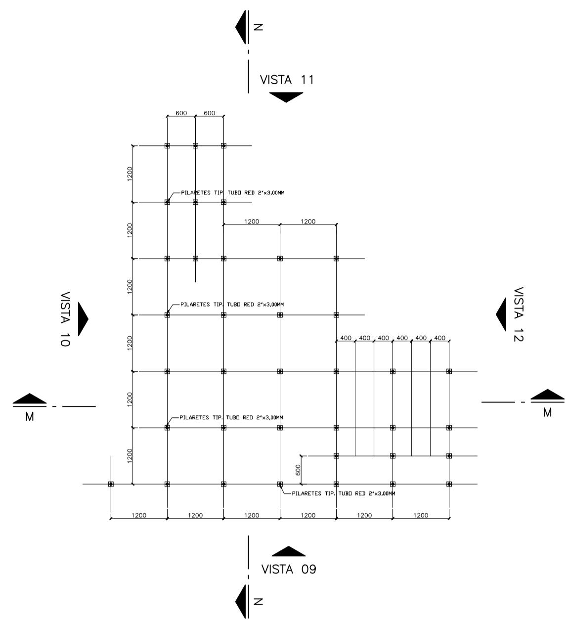
CONJUNTO 03 – Nível 0,00 ESCALA 1:75
