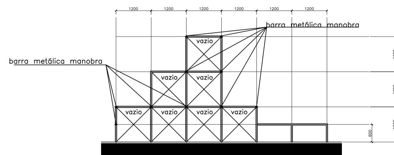
CORTE NN ESCALA 1:75
