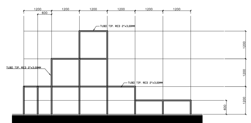
VISTA 12 ESCALA 1:75
