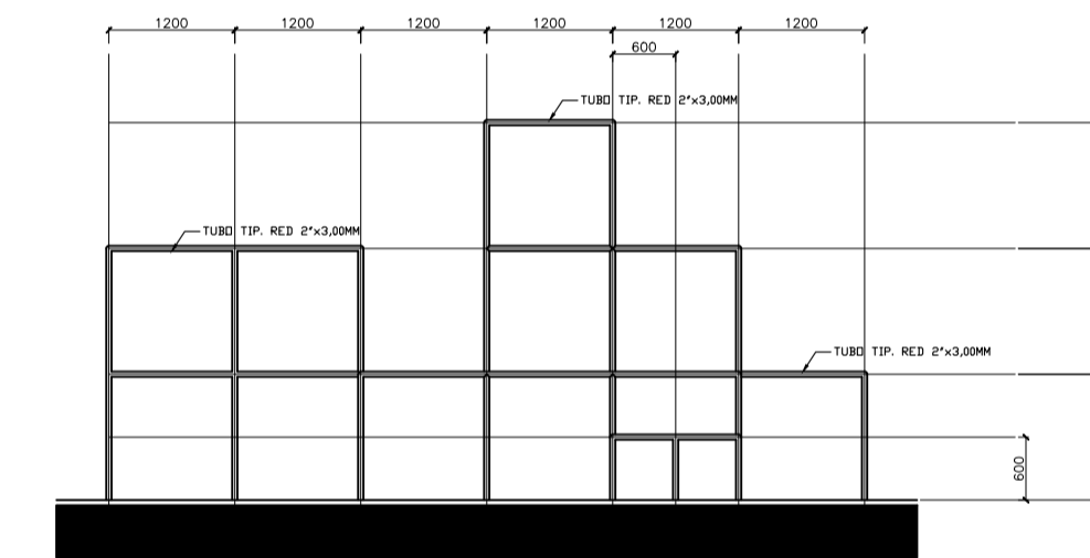
VISTA 11 ESCALA 1:75
