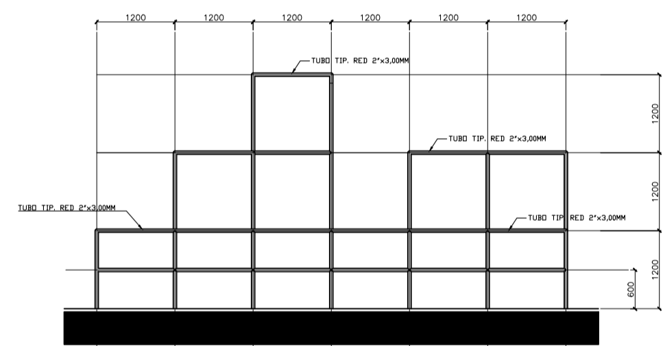
VISTA 09 ESCALA 1:75
