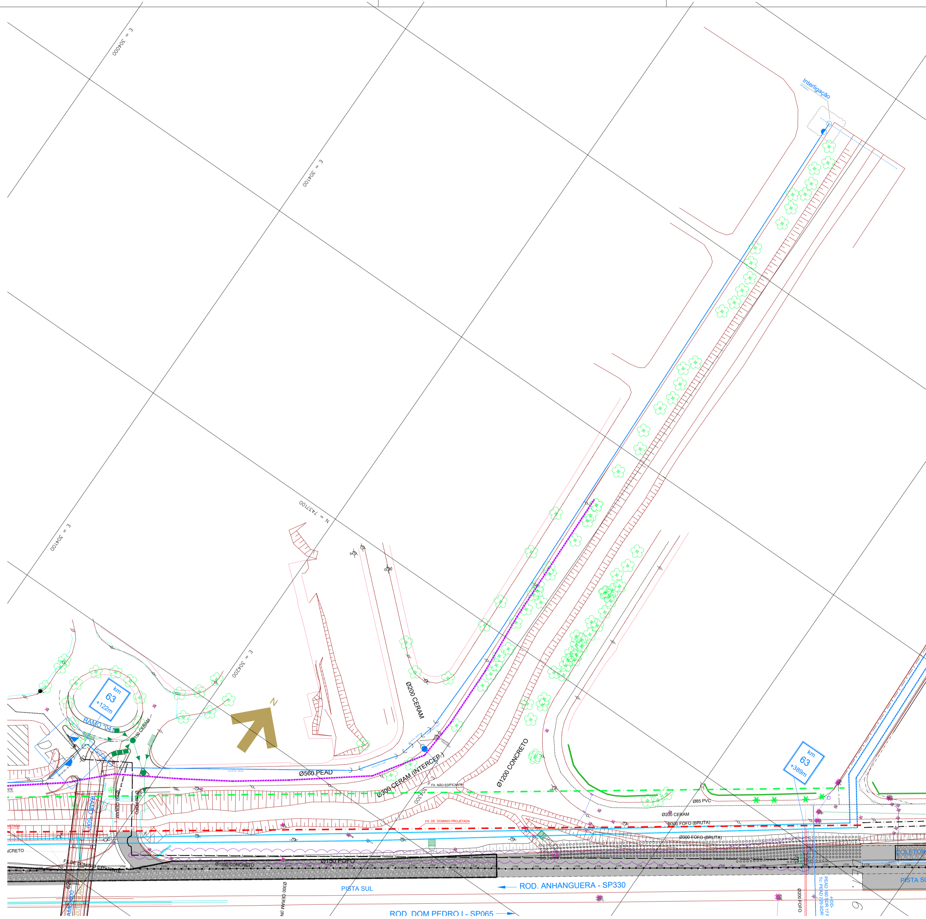
IMPLANTAÇÃO ADUTORA 150mm - PQ. DA REPRESA EXTENSÃO DA ADUTORA A SER INTALADA DN 250/200 ESC.: 1:50
