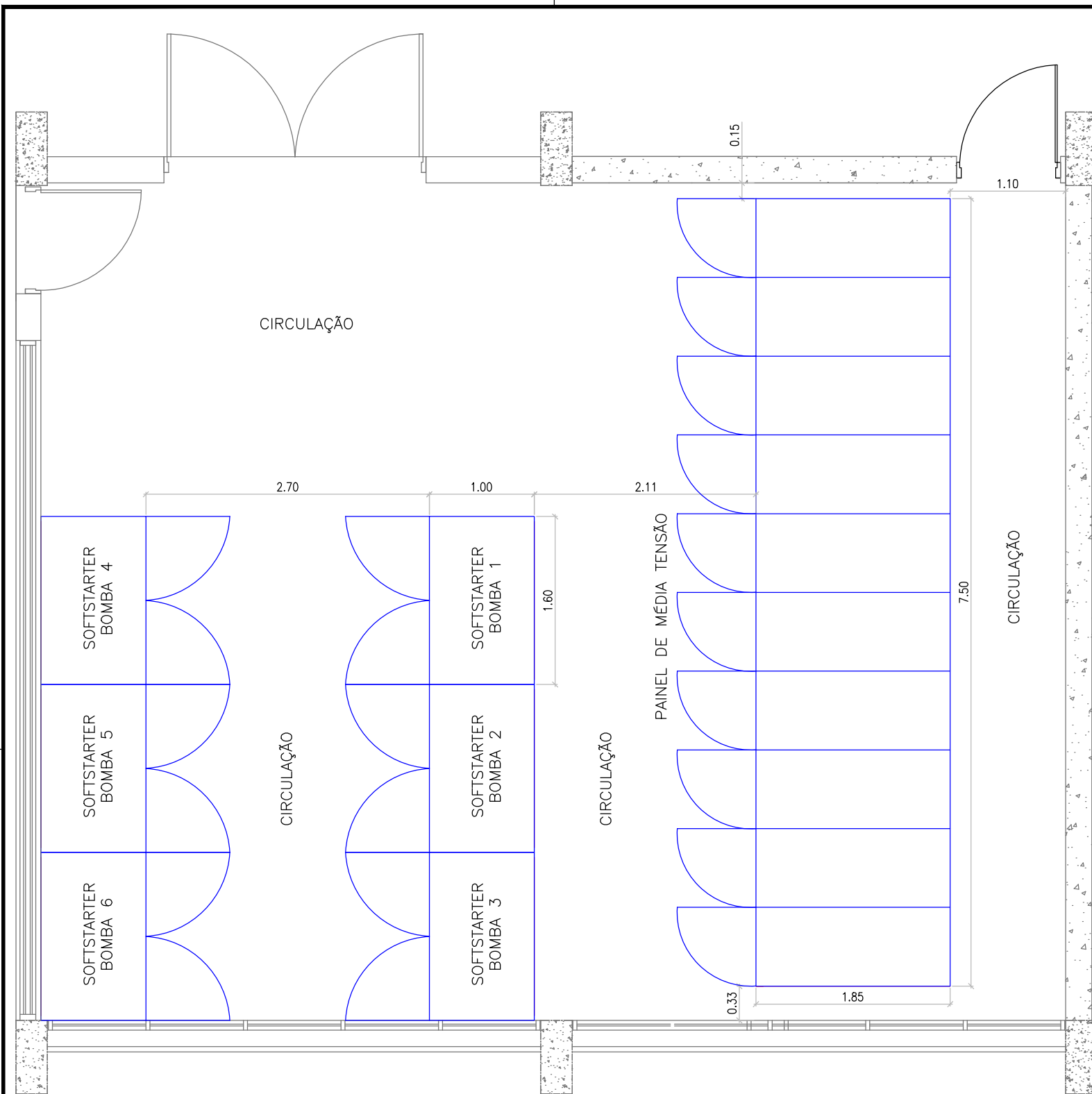
PLANTA-SALA DE PAINÉIS-EEAB RIO JUNDIAI MÍRIM ESCALA 1:50
