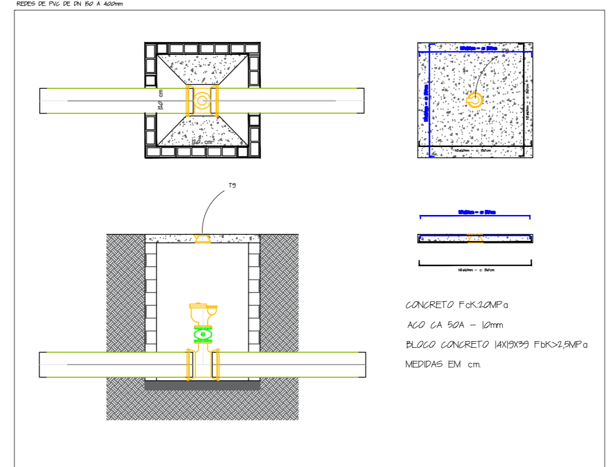
CAIXA DE VALVULA DE MANEIRA ADUTORAS DE DN 150 A 450 mm
