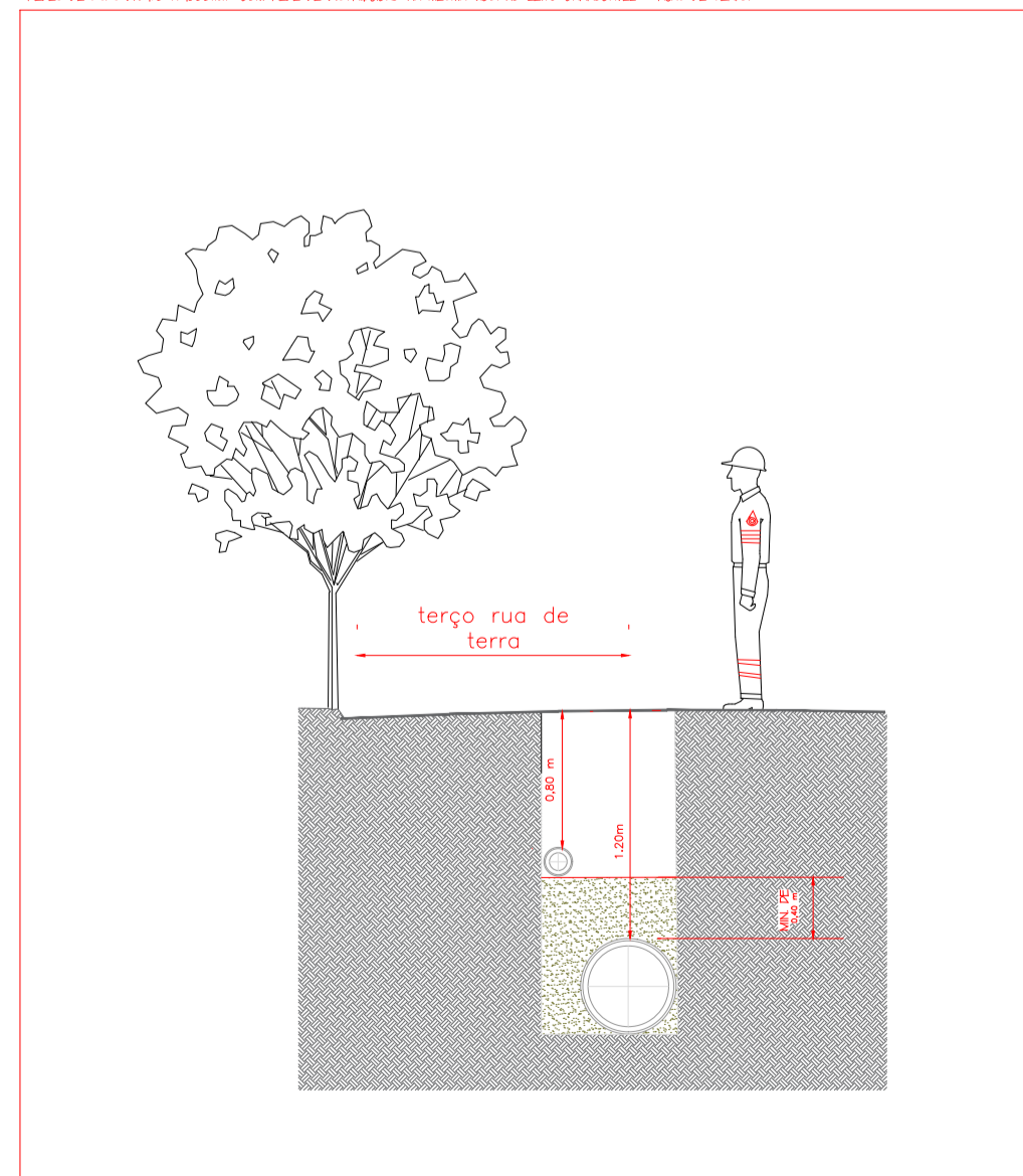
DETALHAMENTO DA(S) V.C.A(S) EM VIAS PÚBLICAS COM 2 REDES REDES DE FIFOS DE 100 A 150MM, COM REDE DE DISTRIBUIÇÃO NA MESMA V.C.A. NO LADO CARROZEL - RUA DE TERRA
