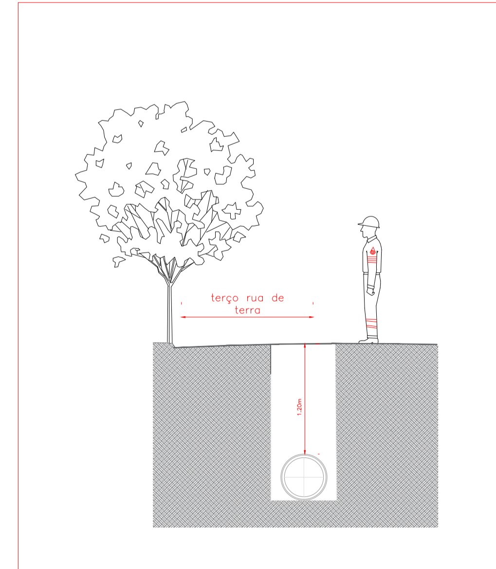
DETALHAMENTO DA(S) V.C.A(S) EM VIAS PÚBLICAS DE TERRA REDES DE FIFOS DE 100 A 150MM, COM REDE DE DISTRIBUIÇÃO NA MESMA V.C.A. NO LADO CARROZEL
