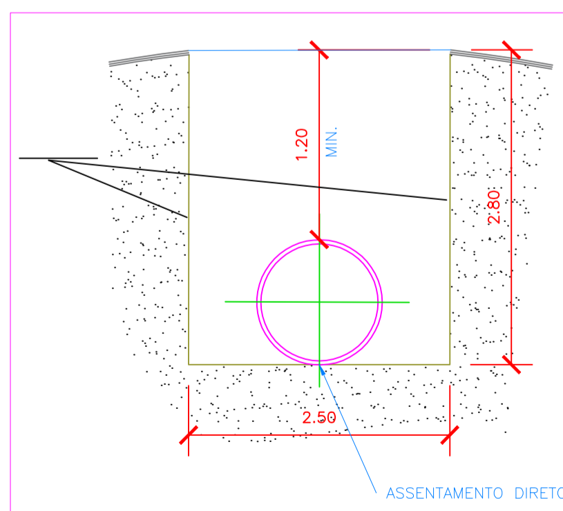
DETALHE TÍPICO DE ABERTURA DE VALA
