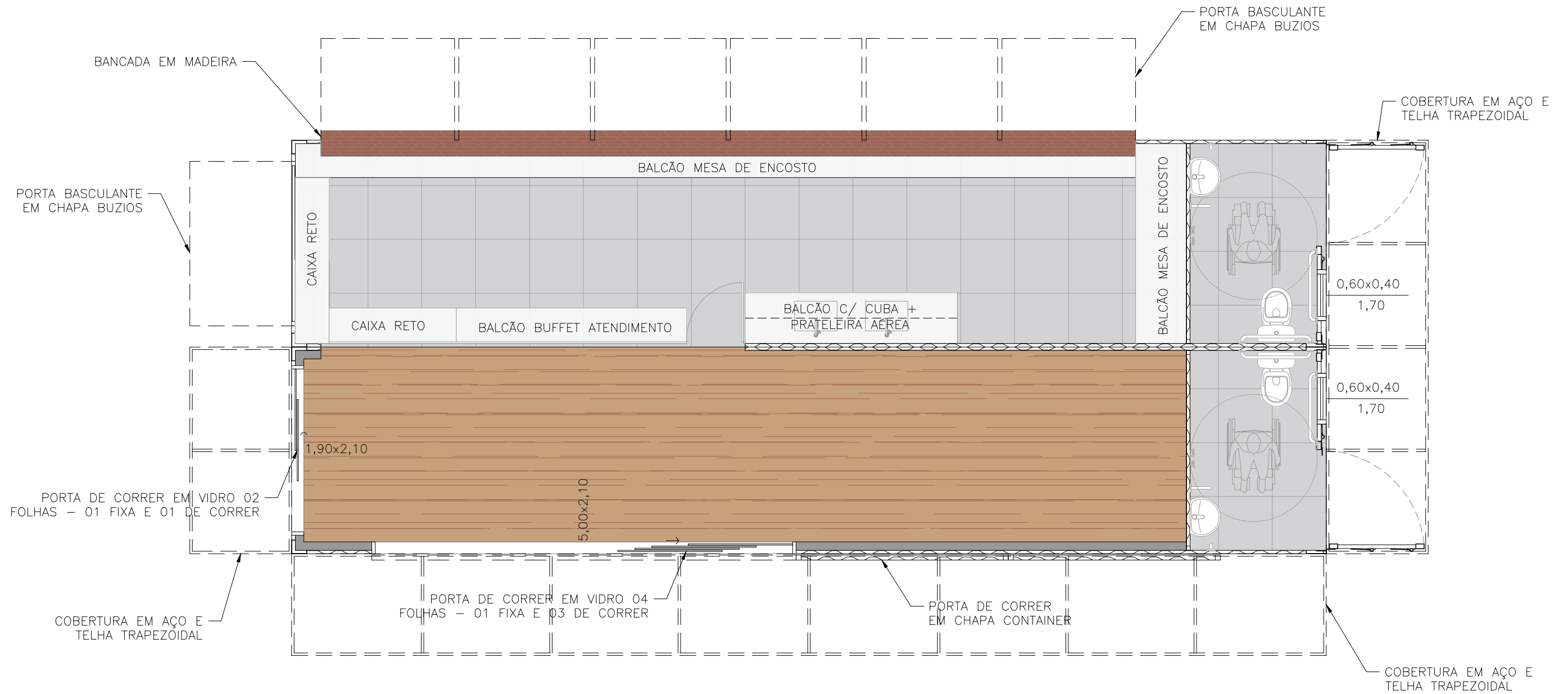
1 PLANTA BAIXA - BAR DA PRAIA ESCALA 1:50
