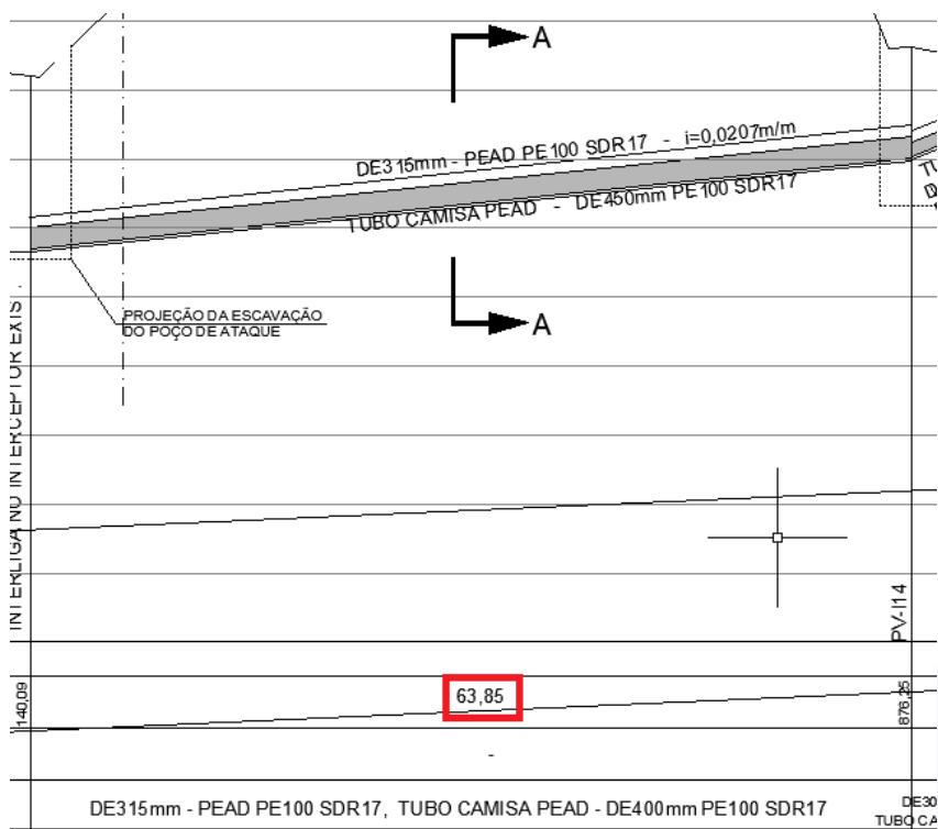
Figura 1-Extensão da travessia prevista em projeto
